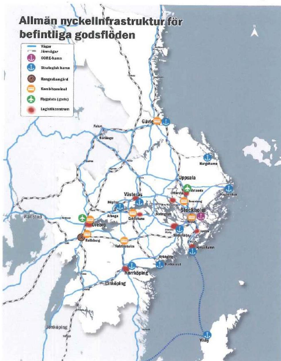
Figur 10. Allmän nyckelinfrastruktur för befintliga godsflöden i Stockholm-Mälarenregionen.
