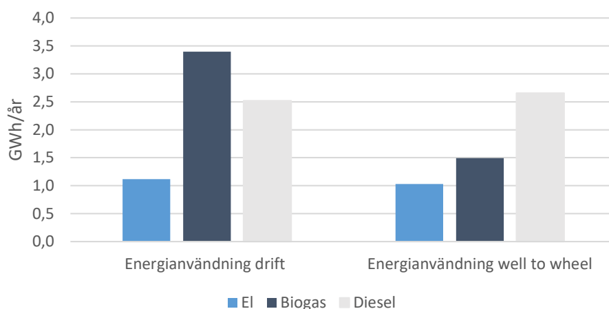
Figur 3. Energianvändning för linje 5 per drivmedel vid drift respektive ur ett well-to-wheel-perspektiv.
